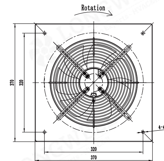
LWAD3G250ZB-7MKW-08(吹风)
