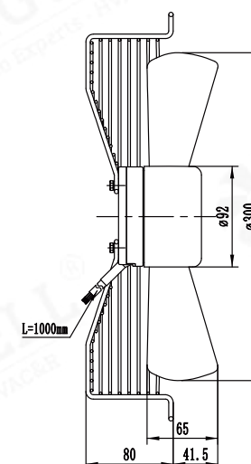
LWAD3G300ZS-5PKW-05(吸风)
