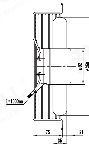
LWAD3G250ZS-7MKW-07(吸风)
