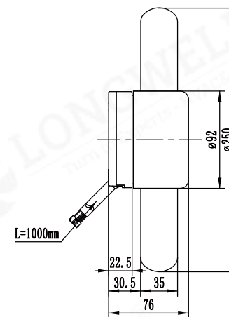
LWAD3G250ZS-7MEW-05(吸风)
