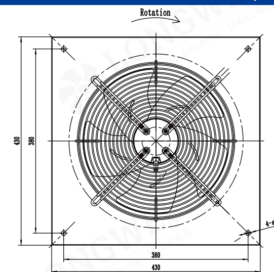
LWAD3G300ZB-5PKW-06(吹风)
