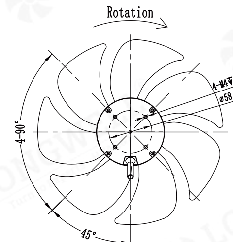
LWAD3G250ZB-7MNV-04(吹风)
