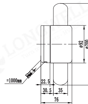
LWAD3G200ZS-7MEW-05(吸风)
