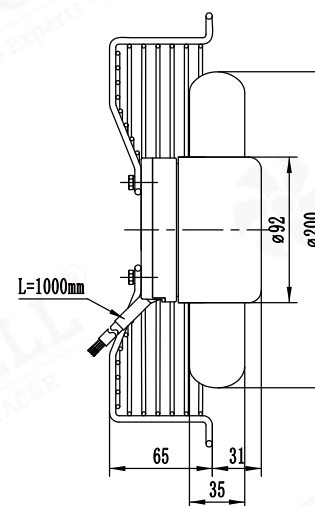
LWAD3G200ZS-7MGW-07(吸风)
