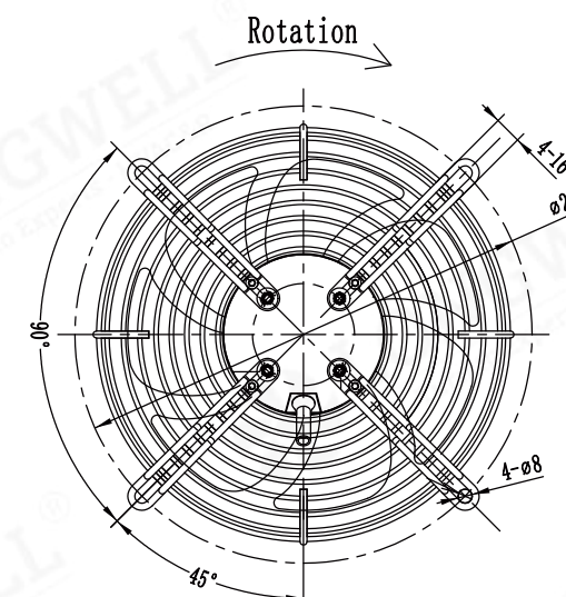
LWAD3G200ZB-7MEW-06(吹风)
