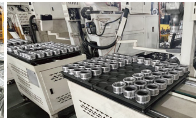
自动焊接机
