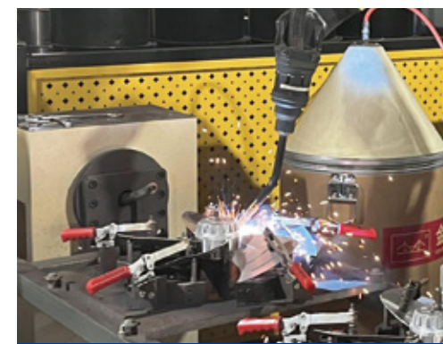
自动焊接
