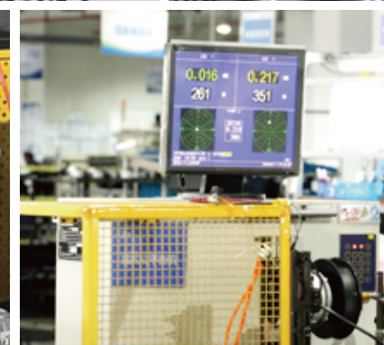
平衡机
