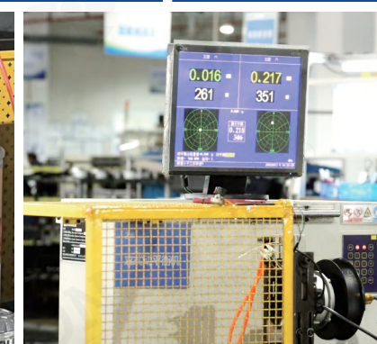
平衡机
